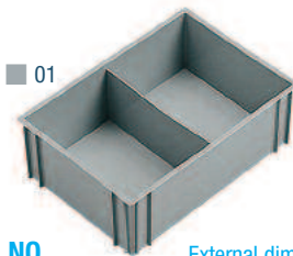
ORD. NO. External dim. mm F PP 4551 00 01 256x176x90 h Standard colour
